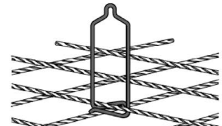
Bild 10: SPA-B Schenkel zusammendrücken und drehend am unteren Mattenstab anclicken.
