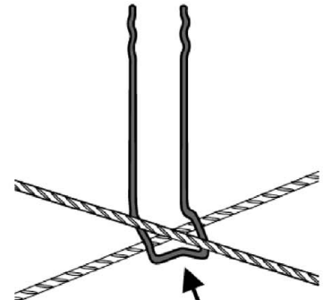
Bild 7: SPA-A am Mattenkreuz festklemmen.
